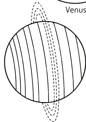
Uranus
