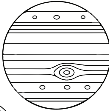
Jupiter
